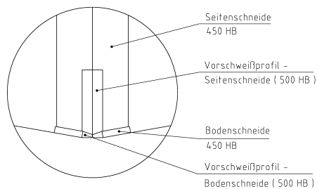
Verstärkte Boden- und Seitenschneden
